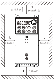
图 2-1 安装的间隔距离
