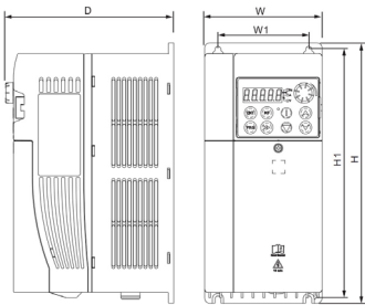
图 C-9 框架 C 安装尺寸
