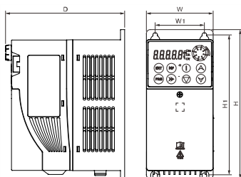
图 C-7 框架 A 安装尺寸
