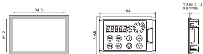
图 C-6 键盘底座安装尺寸 (单位: mm)
