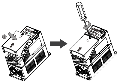
图 C-4 端子盖的安装
