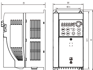
图 C-8 框架 B 安装尺寸
