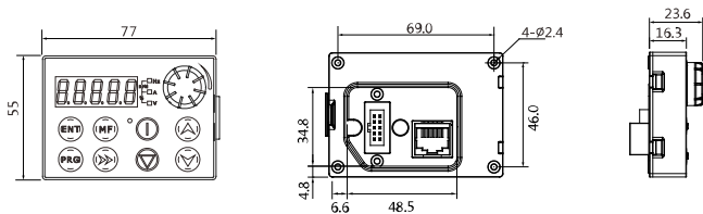
图 C-5 键盘安装尺寸 (单位: mm)
