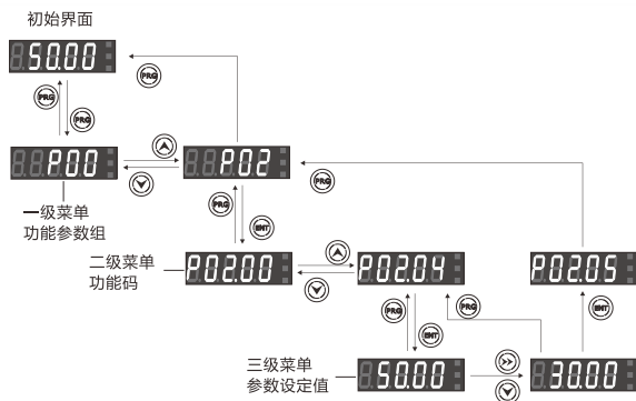
图 3-2 参数查询与修改流程
