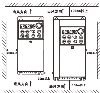
图 2-3 两台变频器左右安装
