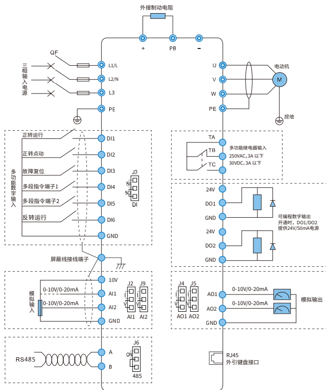
图 2-6 S100 系列变频器系统配线图
