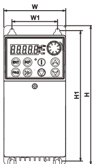
图 2-4 壁挂式安装示意图
